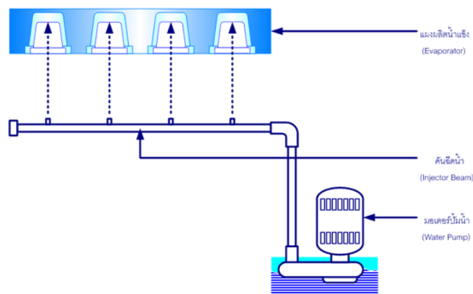
ภาพที่ 7-5 การผลิตน้ำแข็งยูนิตก้อนตัน หรือน้ำแข็งถ้วย ในขั้นตอนการทำน้ำให้แข็ง
