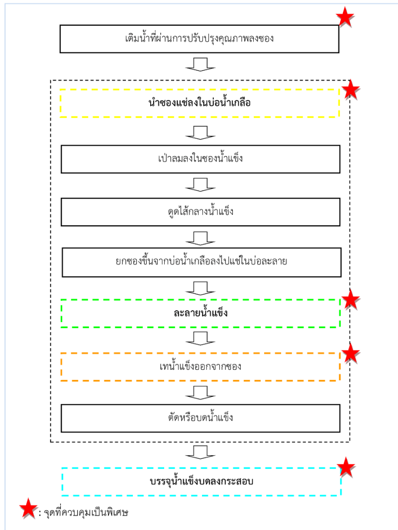
ภาพที่ 7-1 แผนภูมิแสดงขั้นตอนการผลิตน้ำแข็งของและน้ำแข็งบด
