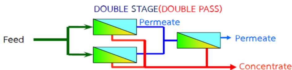
ภาพที่ 4-14 น้ำกรองที่ได้จากขั้นตอนแรกถูกส่งไปยังขั้นตอนที่ 2 เพื่อขจัดสารละลายเพิ่มขึ้น เรียกว่า Double state
